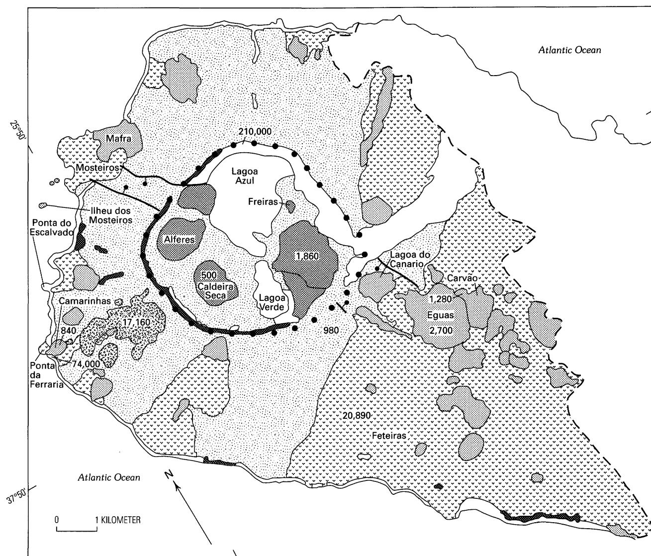
Figure 3 (above and facing page). Generalized geologic map of Sete Cidades volcano.
